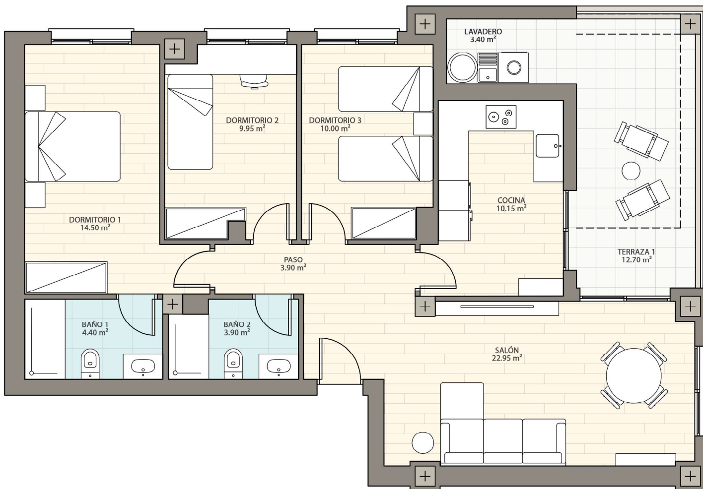
(Plano Distribución 1)
