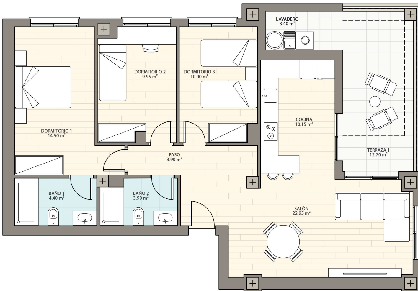
(Plano Distribución 2)
